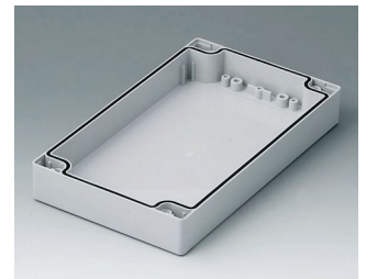
C1122002 Coquille 120, avec joint PC (UL 94 HB) gris clair RAL 7035 200x120x30mm
