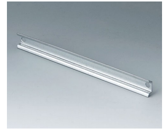
C7113087 Barrette normalisée, type TH 15 Acier 144x15x5,5mm
