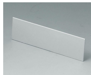
A9109111 Plaque avant / arrière V, O 155 Aluminium anodisé mat 81,9x23,6x1mm
