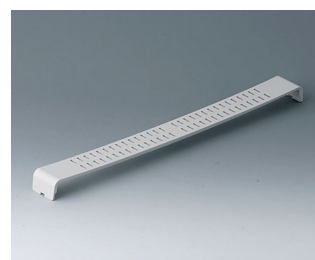
A0126370 Élément d'aération, avec fentes ABS (UL 94 HB) gris blanc RAL 9002
