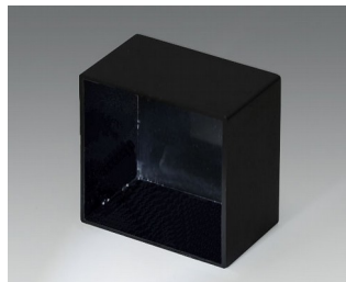
A8032208 BOITIER VIDE POUR MODULES, Vers. III PA 66 (UL 94 V-2) noir RAL 9005 32,4x32,4x20mm
