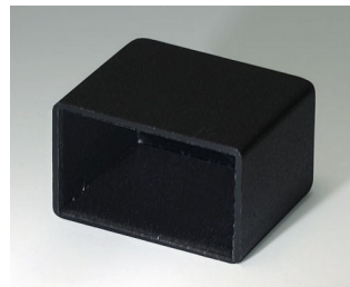
A8021178 BOITIER VIDE POUR MODULES, Vers. III PA 66 (UL 94 V-2) noir RAL 9005 21,3x13,3x17,7mm
