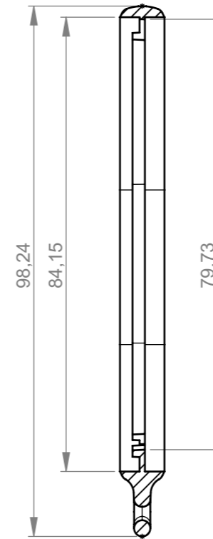
Schnitt A-A
