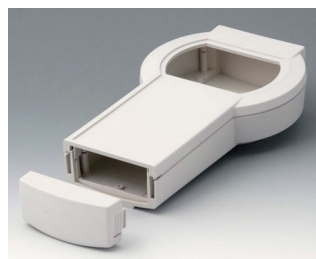
A9079207 DATEC-CONTROL L, исп. I АБС (UL 94 HB) белый RAL 9002 266x144x60mm IP 54 opt.
