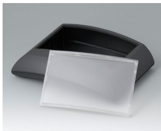
B7020149 ERGO-CASE L, плоский АБС (UL 94 HB) черный RAL 9005 150x200x54mm IP 40
