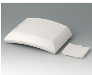
B7020107 ERGO-CASE L, плоский АБС (UL 94 HB) белый RAL 9002 150x200x54mm IP 54 opt.
