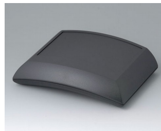
B7020209 ERGO-CASE L, плоский АБС (UL 94 HB) черный RAL 9005 150x200x54mm IP 54 opt.
