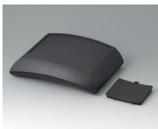
B7020109 ERGO-CASE L, плоский АБС (UL 94 HB) черный RAL 9005 150x200x54mm IP 54 opt.
