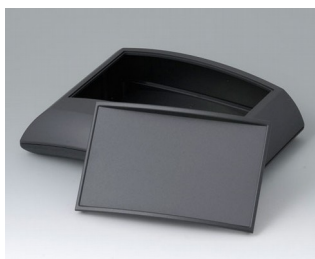
B7020239 ERGO-CASE L, плоский АБС (UL 94 HB) черный RAL 9005 150x200x54mm IP 40
