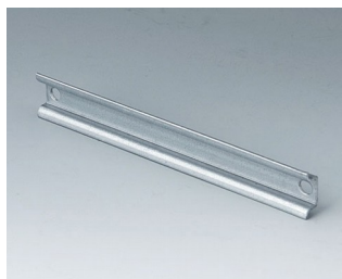
C7112087 DIN-рейка TH 15 Сталь 108x15x5,5mm
