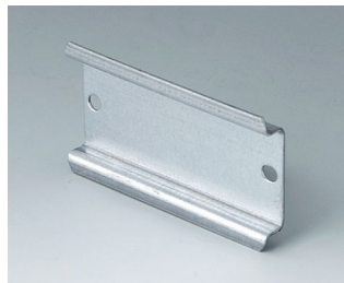
C7110077 DIN-рейка TH 35 Сталь 66x35x7,5mm
