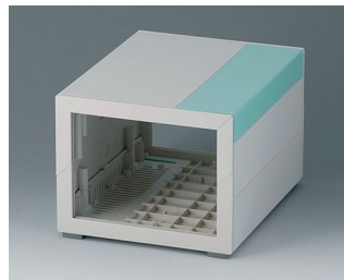
B2213215 MEDITEC E 160, без ручки АБС (UL 94 HB) белый RAL 9002 160x200x124mm IP 40
