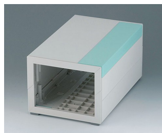
B2212215 MEDITEC E 220, без ручки АБС (UL 94 HB) белый RAL 9002 160x260x124mm IP 40
