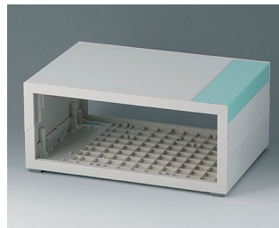
B2211215 MEDITEC D 160, без ручки ABC (UL 94 HB) белый RAL 9002 290x200x124mm IP 40
