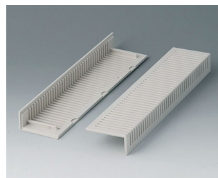
B2021007 Угловые накладки 220, с вентиляцией АБС (UL 94 HB) белый RAL 9002
