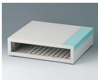
B2210005 MEDITEC D 220, без ручки АБС (UL 94 HB) белый RAL 9002 290x260x74mm IP 40
