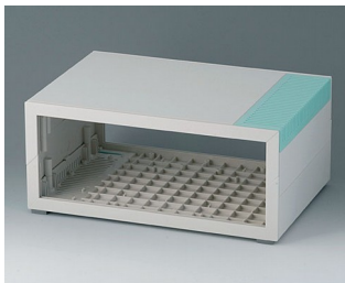
B2211205 MEDITEC D 160, без ручки ABC (UL 94 HB) белый RAL 9002 290x200x124mm IP 40
