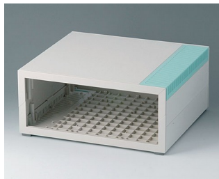
B2210205 MEDITEC D 220, без ручки ABC (UL 94 HB) белый RAL 9002 290x260x124mm IP 40
