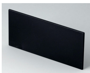
B6132221 Лицевая панель ПФО (UL 94 V-0) черный RAL 9005 91,6x43,5x2mm
