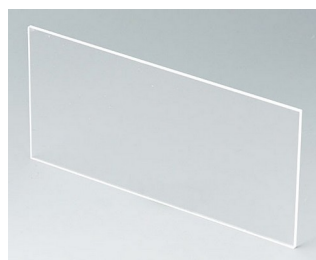
B6143331 Лицевая панель Акриловое стекло прозрачный 139,2x67,3x2mm
