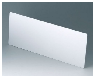
A0336370 Лицевая / задняя панель 63 HP 3 U Алюминий матово-анодированный 357,8x135,2x2mm
