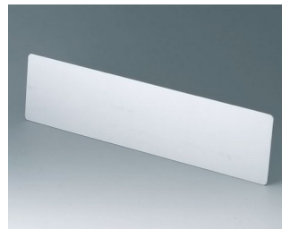
A0326370 Лицевая / задняя панель 63 HP 2 U Алюминий матово-анодированный 357,8x90,7x2mm
