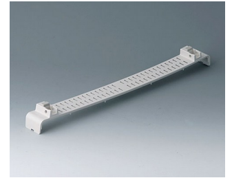
A0146370 Вставка с ножками, с вентиляционными отверстиями АБС (UL 94 HB) белый RAL 9002
