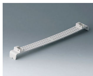
A0146370 Вставка с ножками, с вентиляционными отверстиями АБС (UL 94 HB) белый RAL 9002
