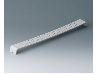
A0126370 Вставка, с вентиляционными отверстиями АБС (UL 94 HB) белый RAL 9002
